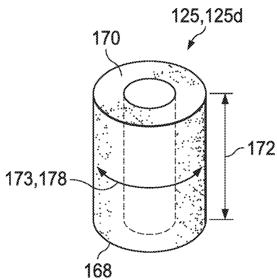
FIG. 7D
