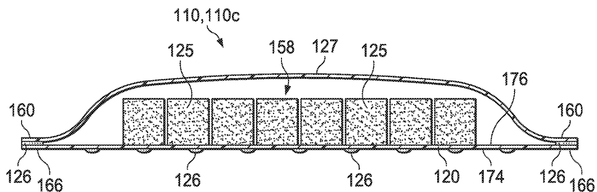
FIG. 3C
