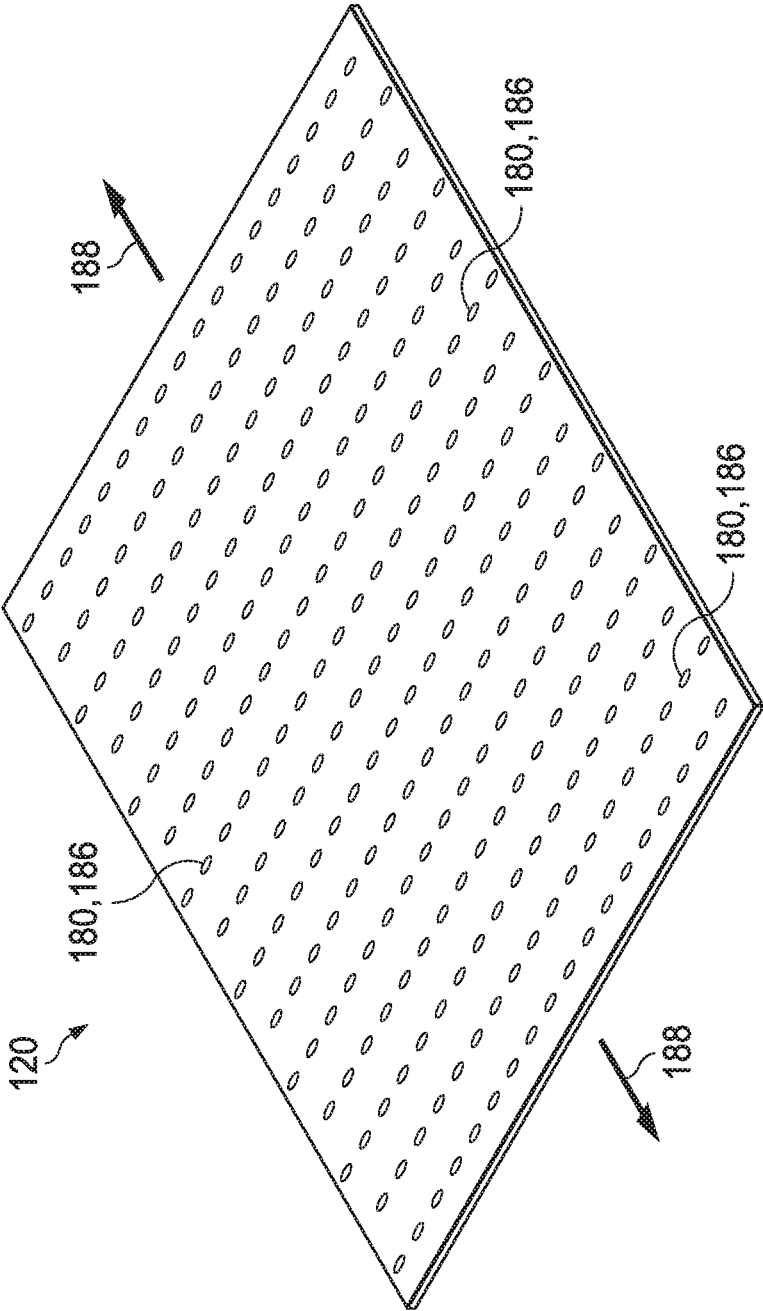
FIG. 10B
