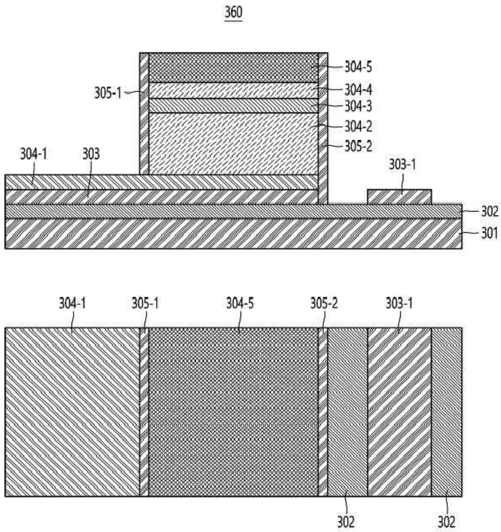
도면3f
