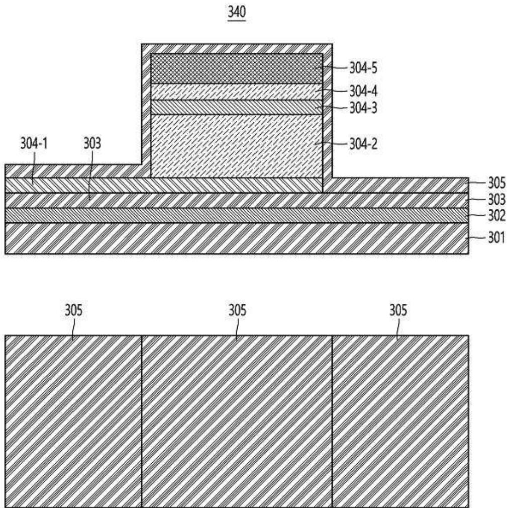
도면3d
