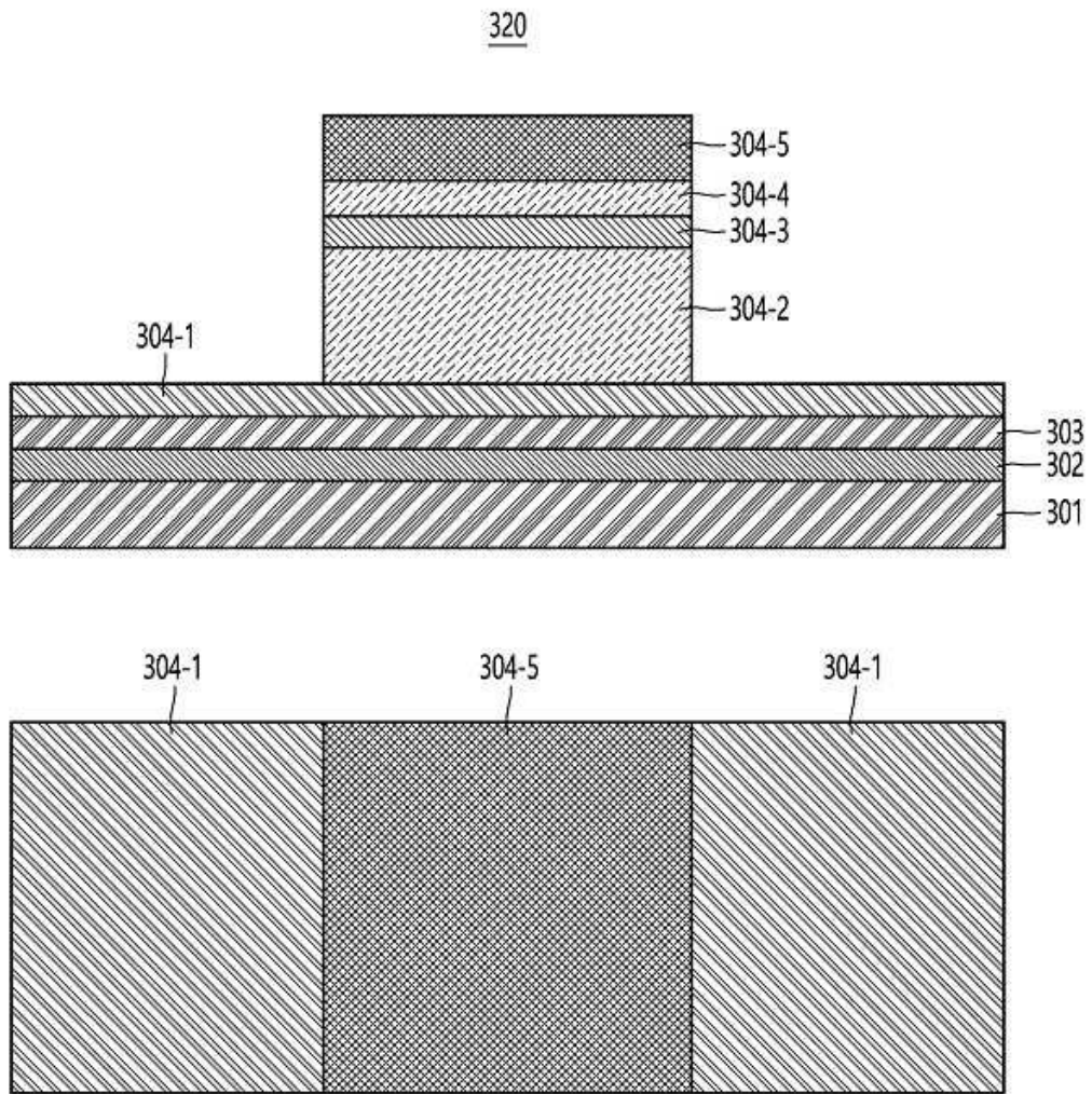
도면 3b
