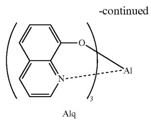
Alq
