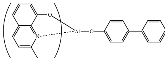
Balq
