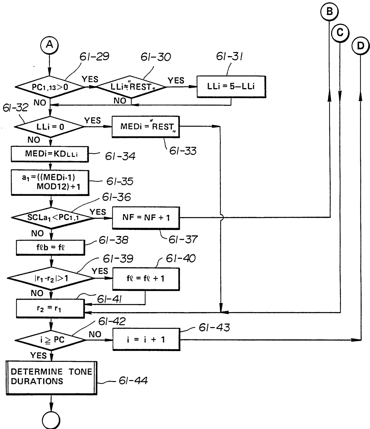
FIG. 61B GENERATE ARPEGGIO
