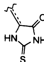
2-thioxo-4-imidazolidinedione
