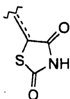
2,4-thiazolidinedione
