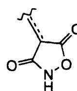
isoxazolidinedione
