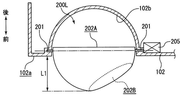
(B) 第 2 状態 (A-A 断面図)
