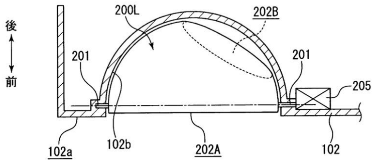
(A) 第 1 状態 (A-A 断面図)
