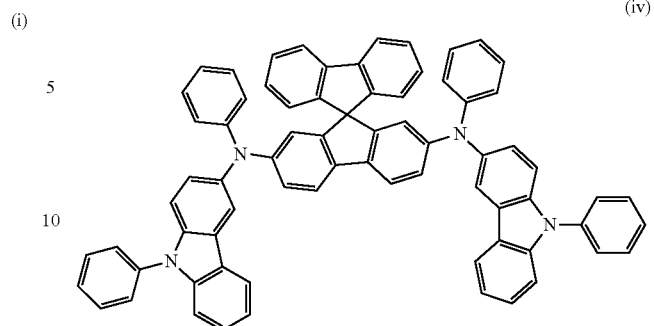
PCA2SF
