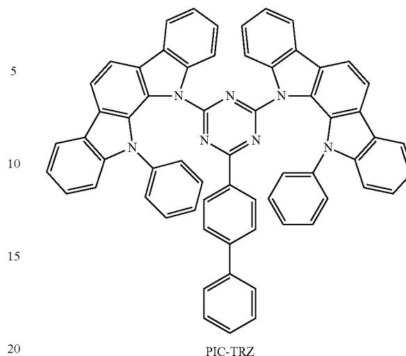
PIC-TRZ
