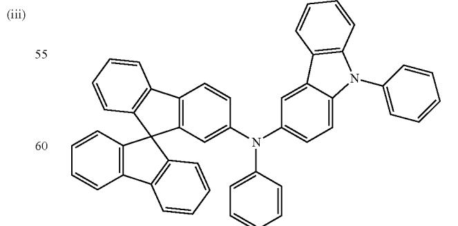
PCASF
