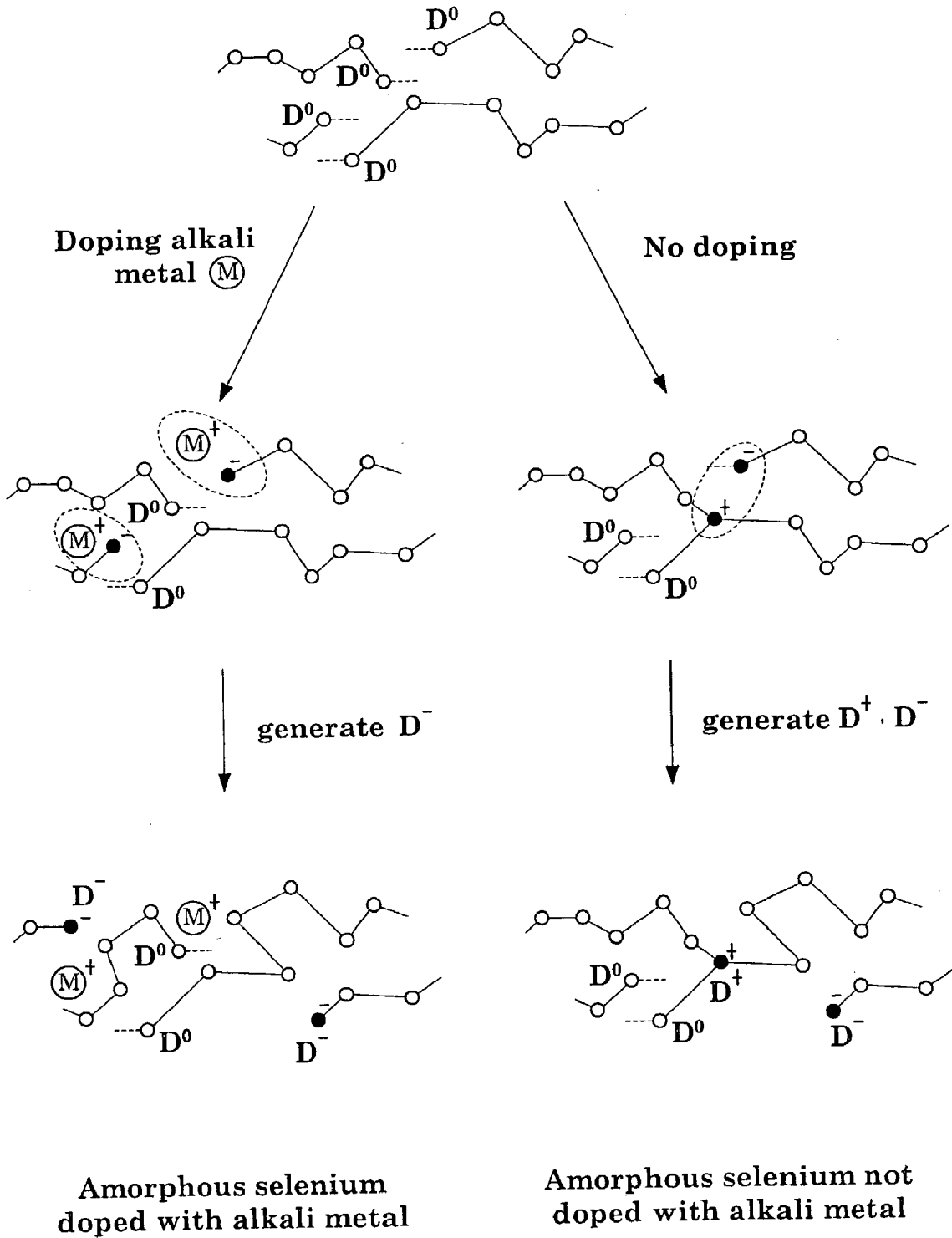
Fig.2B(PRIOR ART)
