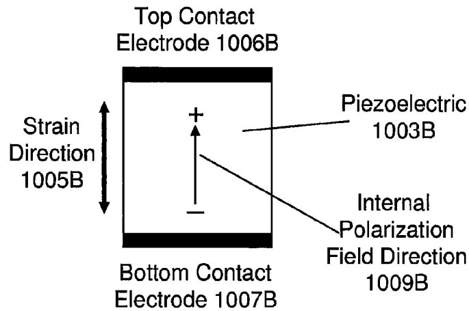
Simple Piezoelectric 1020B
