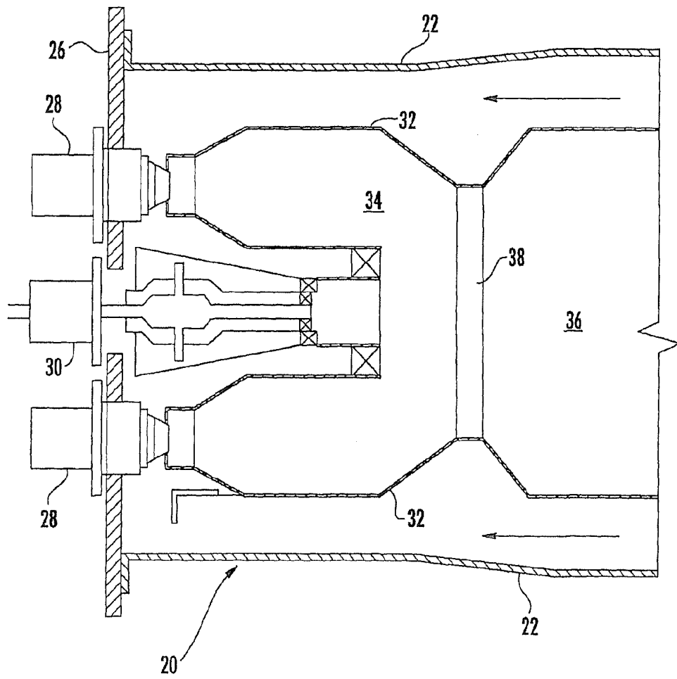
Figur 2 (Stand der Technik)
