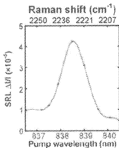
Fig. 6A ATTO 740 C≡N mode
