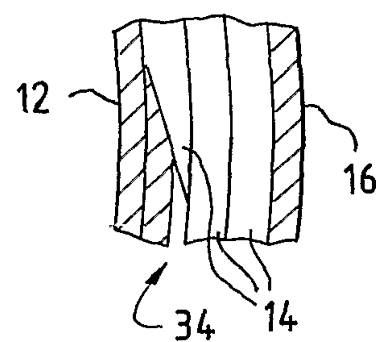
FIG. 6b
