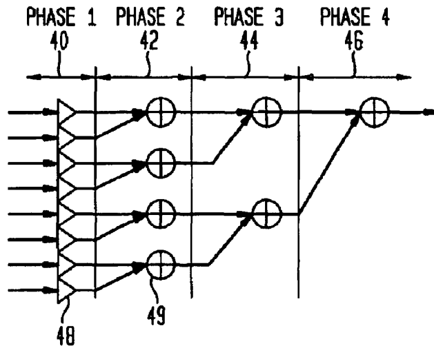
FIG. 6A RADIX-8 DIT FFT ENGINE
