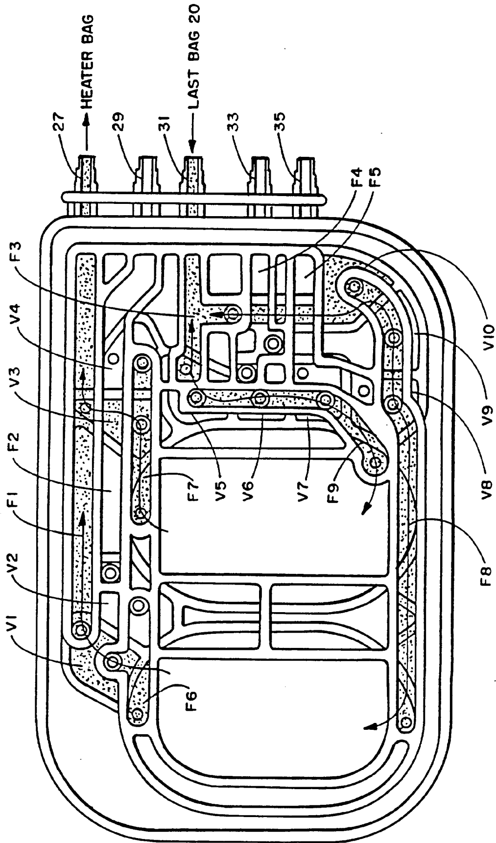
FIG. 35 (LAST DWELL)
