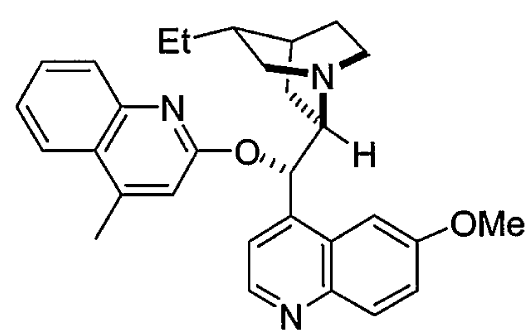
DHQD-MEQ
