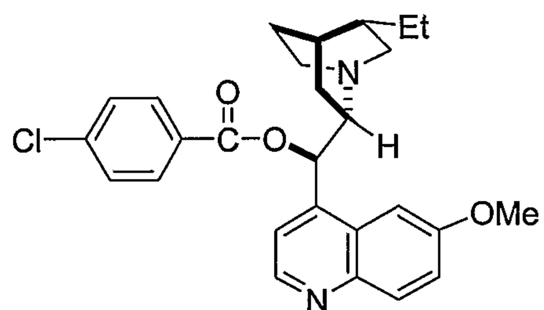
DHQ-CLB
