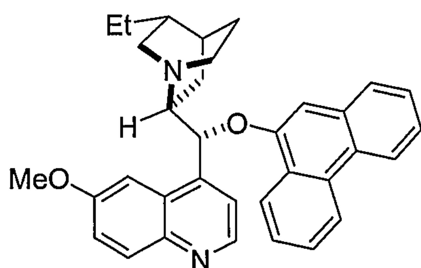
DHQ-PHN
