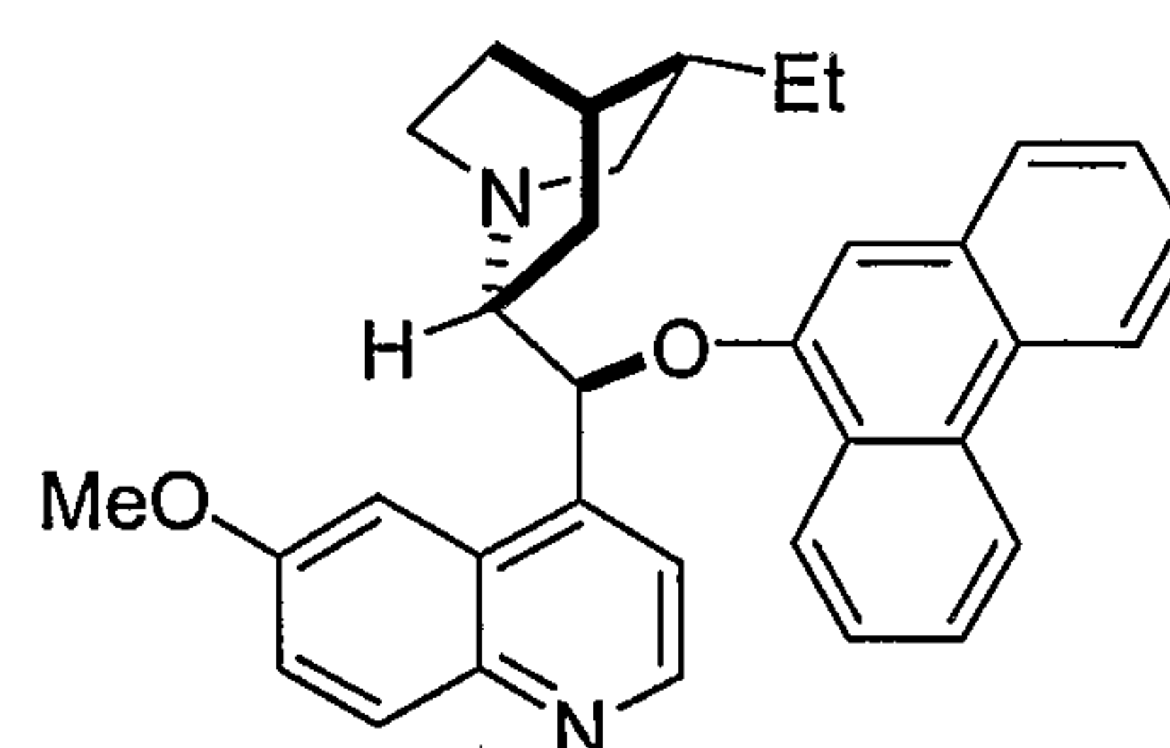
DHQD-PHN
