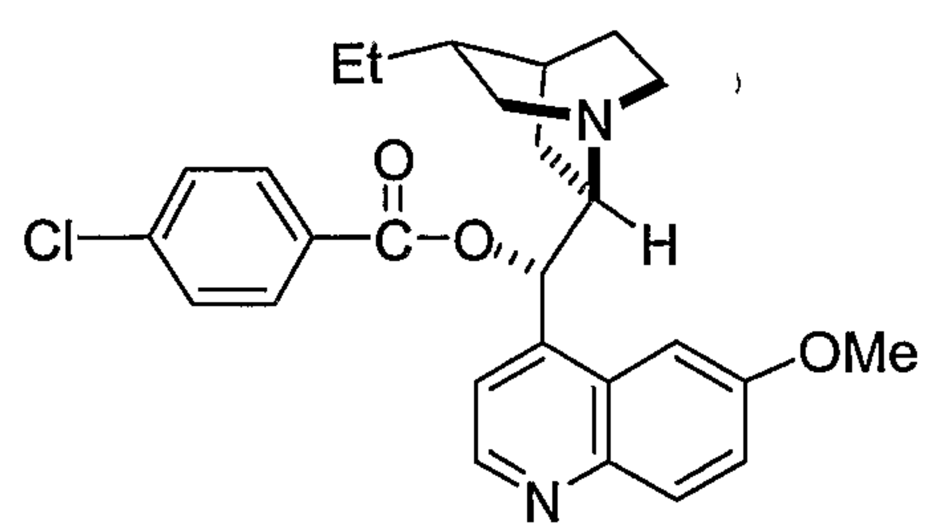
DHQD-CLB
