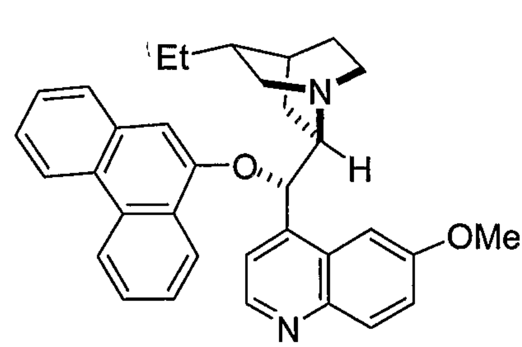
DHQD-AQN
