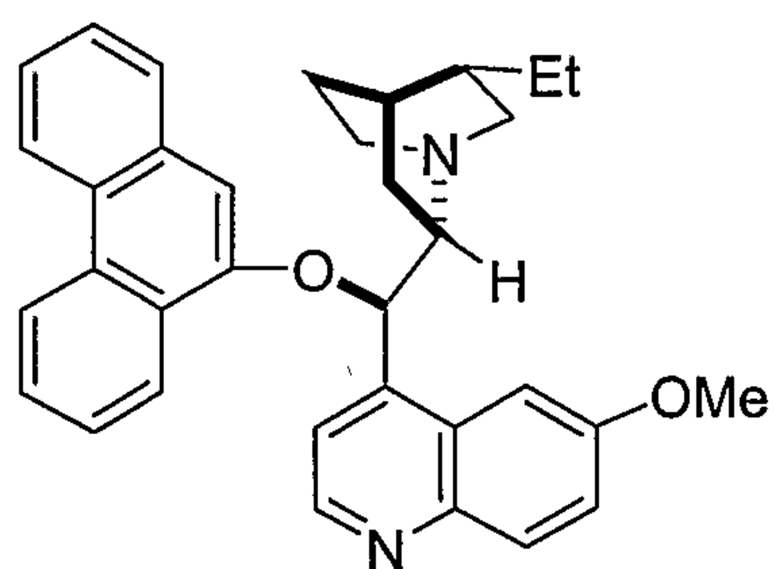
DHQ-AQN
