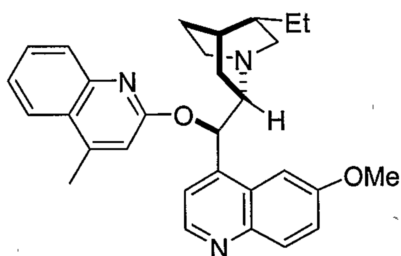
DHQ-MEQ
