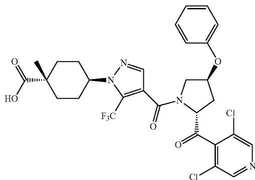
trans-4-(4#(2R,4S)-2#3,5-dichloro-4-pyridinyl)carbonyl)-4-phenoxy-1-pyrrolidinyl)carbonyl)-5-(trifluoromethyl)-1H-pyrazol-1-yl)-1-methylcyclohexanecarboxylic acid
