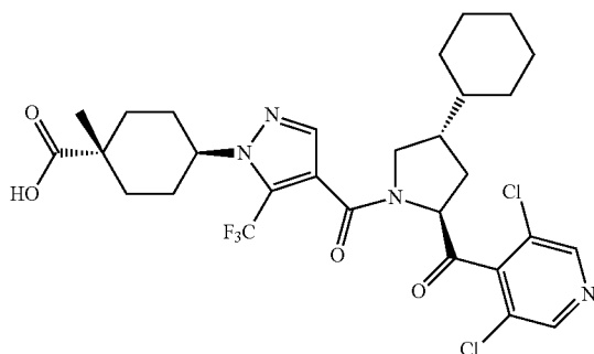
trans-4-(4-(((2S,4S)-4-cyclohexyl-2-(3,5-dichloro-4-pyridinyl)carbonyl)-1-pyrrolidinyl)carbonyl)-5-(trifluoromethyl)-1H-pyrazol-1-yl)-1-methylcyclohexanecarboxylic acid
