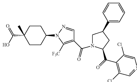
trans-4-(4-(((2S,4R)-2-(3,5-dichloro-4-pyridinyl)carbonyl)-4-phenyl-1-pyrrolidinyl)carbonyl)-5-(trifluoromethyl)-1H-pyrazol-1-yl)-1-methylcyclohexanecarboxylic acid
