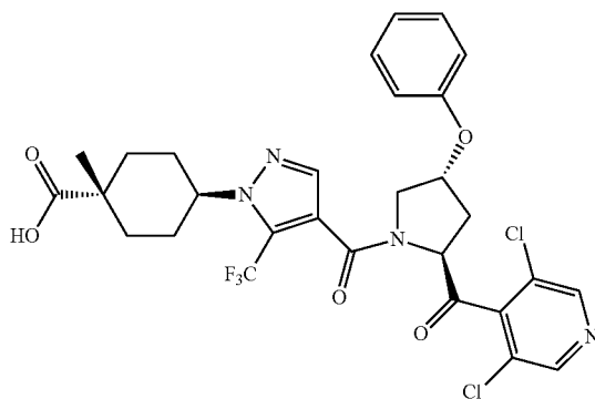
trans-4-(4#(2S,4R)-2#3,5-dichloro-4-pyridinyl)carbonyl)-4-phenoxy-1-pyrrolidinyl)carbonyl)-5-(trifluoromethyl)-1H-pyrazol-1-yl)-1-methylcyclohexanecarboxylic acid
