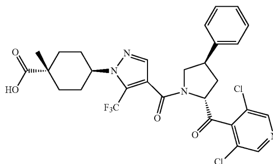
trans-4-(4-(((2R,4R)-2-(3,5-dichloro-4-pyridinyl)carbonyl)-4-phenyl-1-pyrrolidinyl)carbonyl)-5-(trifluoromethyl)-1H-pyrazol-1-yl)-1-methylcyclohexanecarboxylic acid
