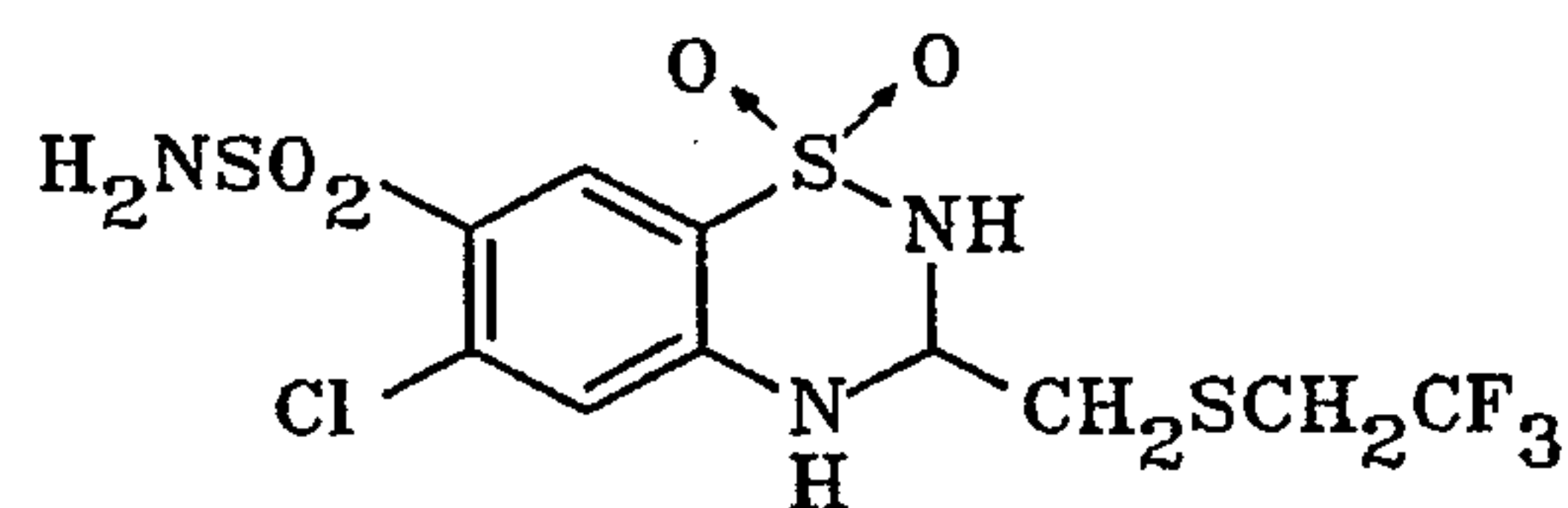
31 epithiazide
