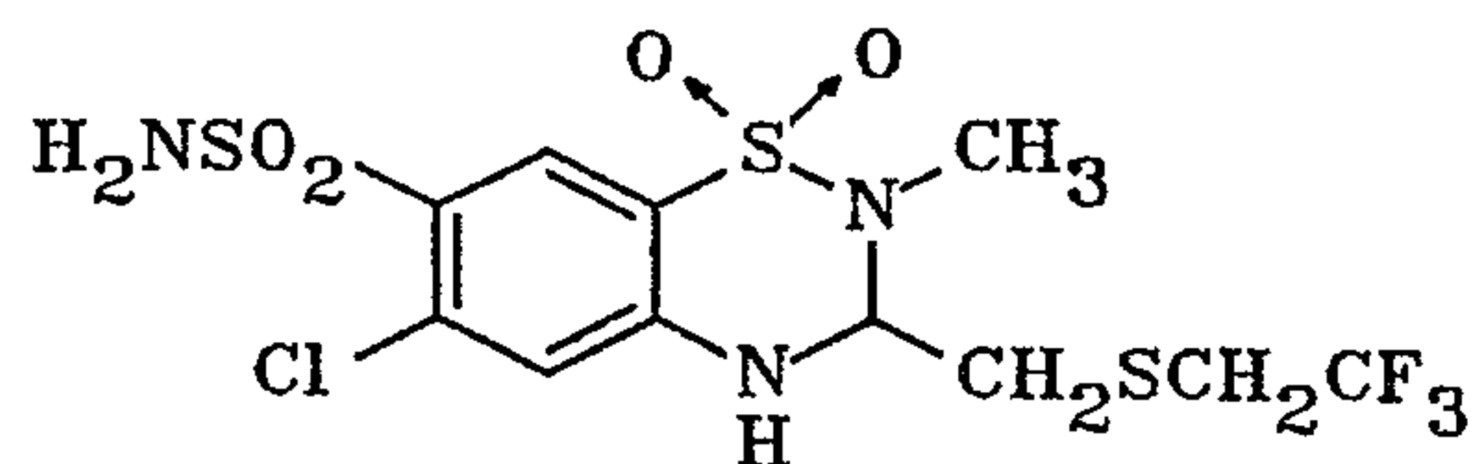
36 polythiazide
