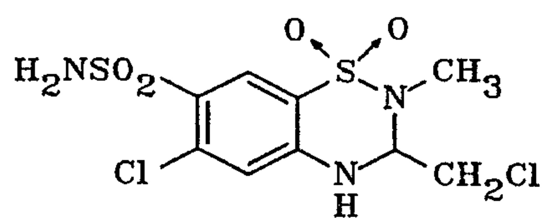
34 methylclothiazide
