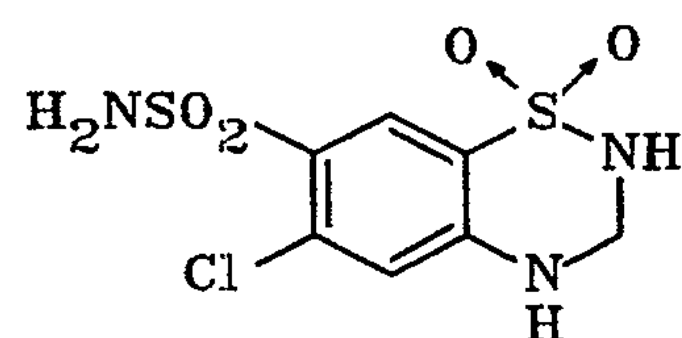
32 hydrochlorothiazide
