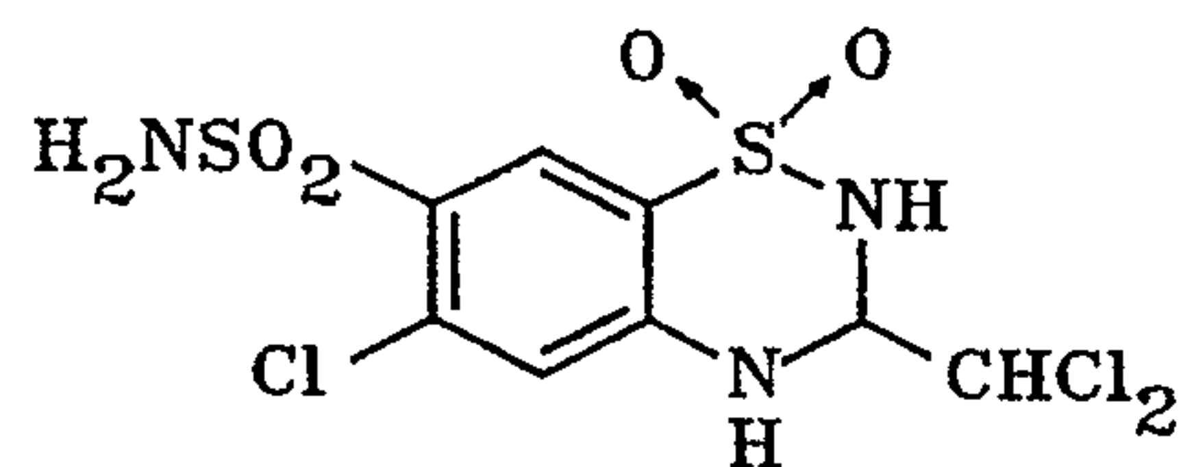
37 trichlormethiazide
