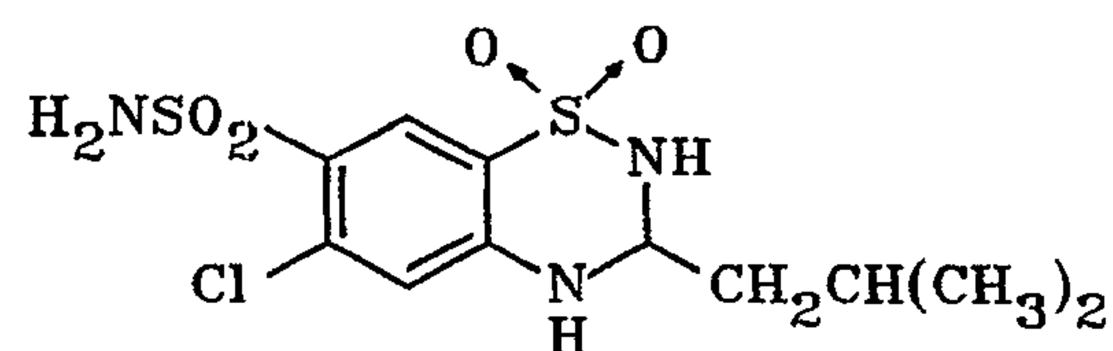
28 buthiazide
