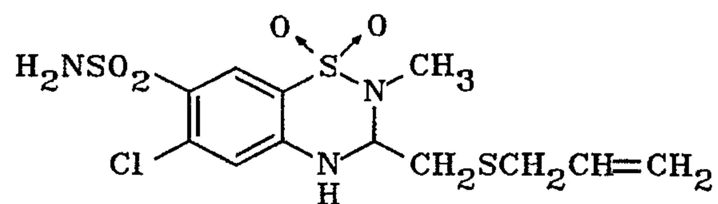
35 methalthiazide
