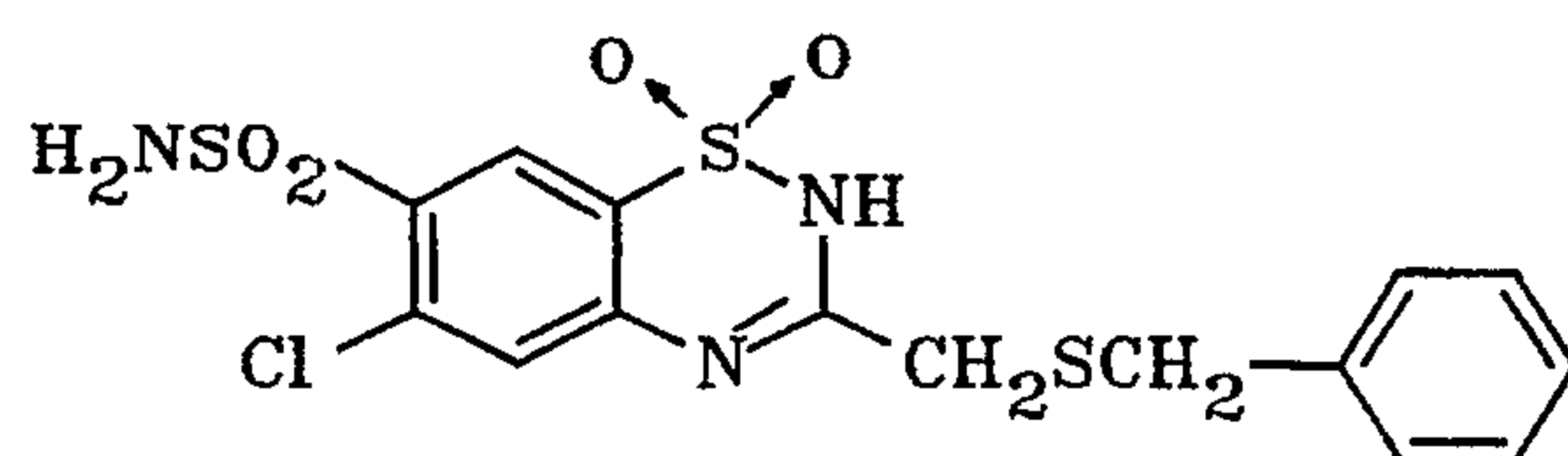
27 benzthiazide
