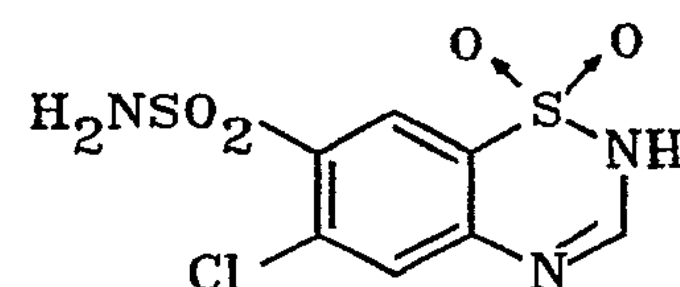
29 chlorothiazide
