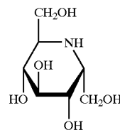
\alpha -Homonojirimycin
