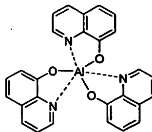
Alq3
