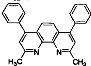
\alpha -NPD
