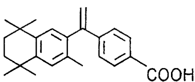
3-METHYL TTNEB
