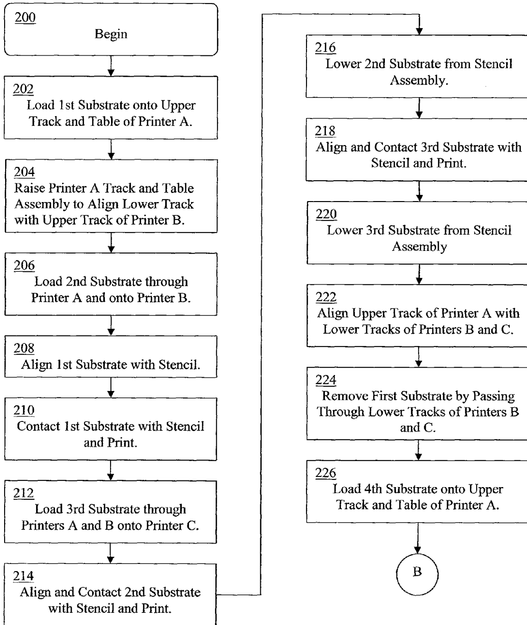
FIG. 27A
