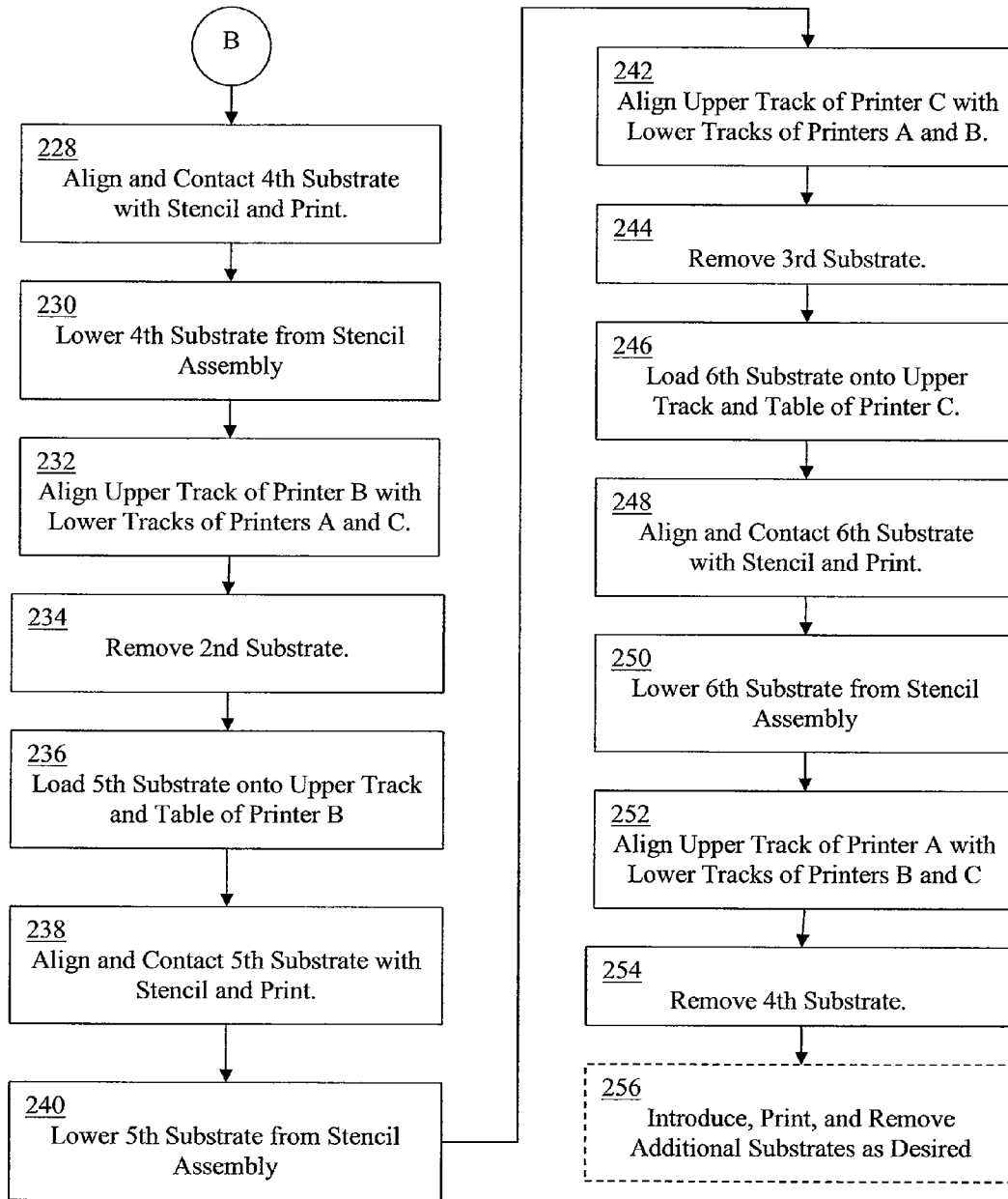
FIG. 27B
