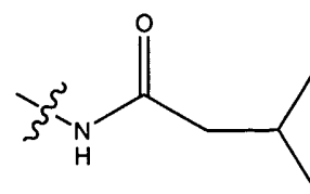
isobutylacetylamine
