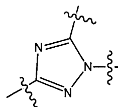
1,3,4-TRIAZOLE
