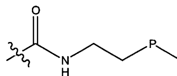
methoxyethylamide
