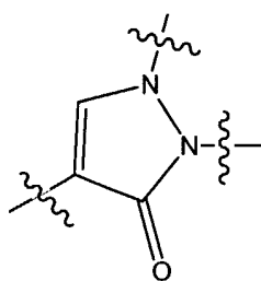
PYRAZOLINONE
