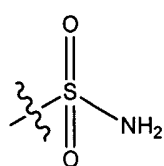
sulfonamide
