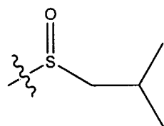
isobutylsulfoxyl
