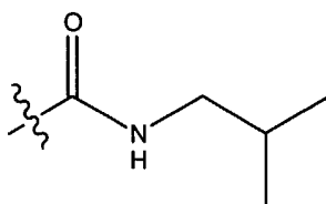
isobutylamide
