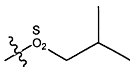
isobutylsulfonyl
