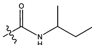
carboxamidobutyl-2-yl
