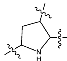
PYRROLIDINE
