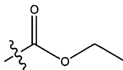
carboethoxy
