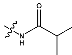
isobutyramido
