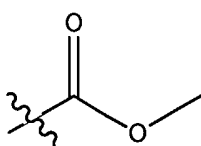
carbmethoxy
