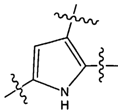
PYRROLE
