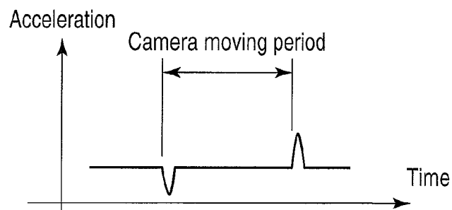
FIG. 2C
