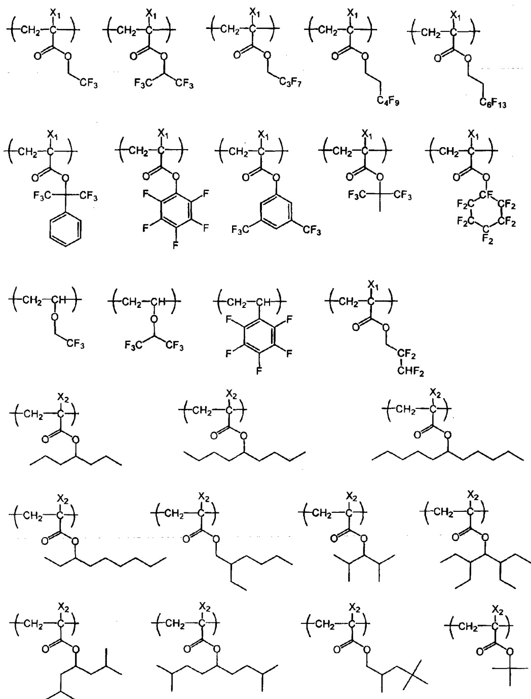
[Chem. 55]
