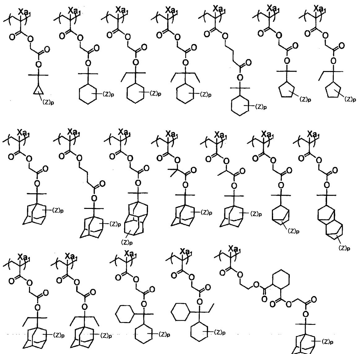
[Chem. 5]
