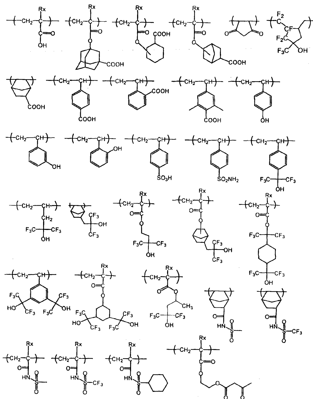
[Chem. 64]
