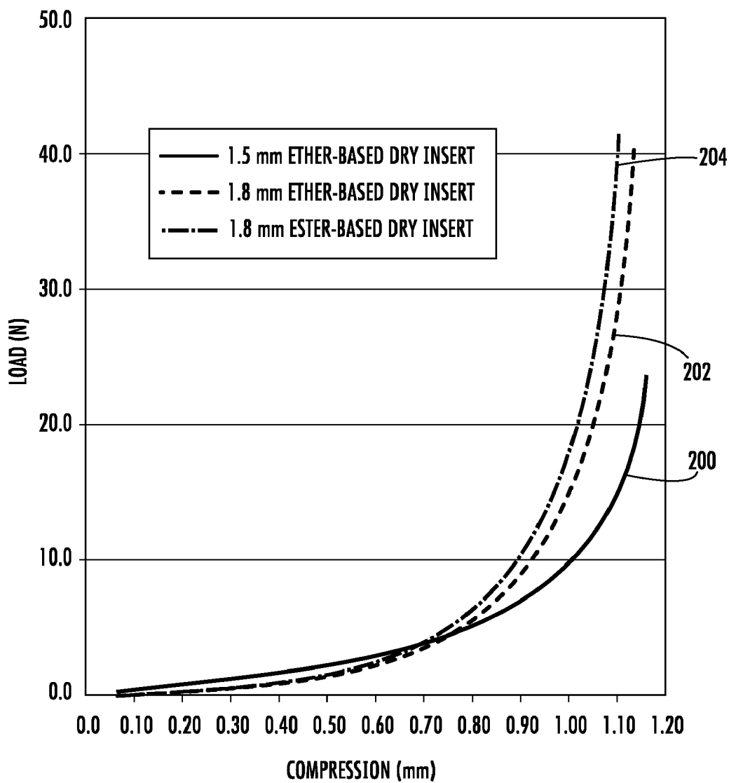
FIG. 2e
