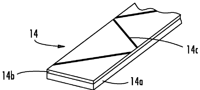
FIG. 2g
