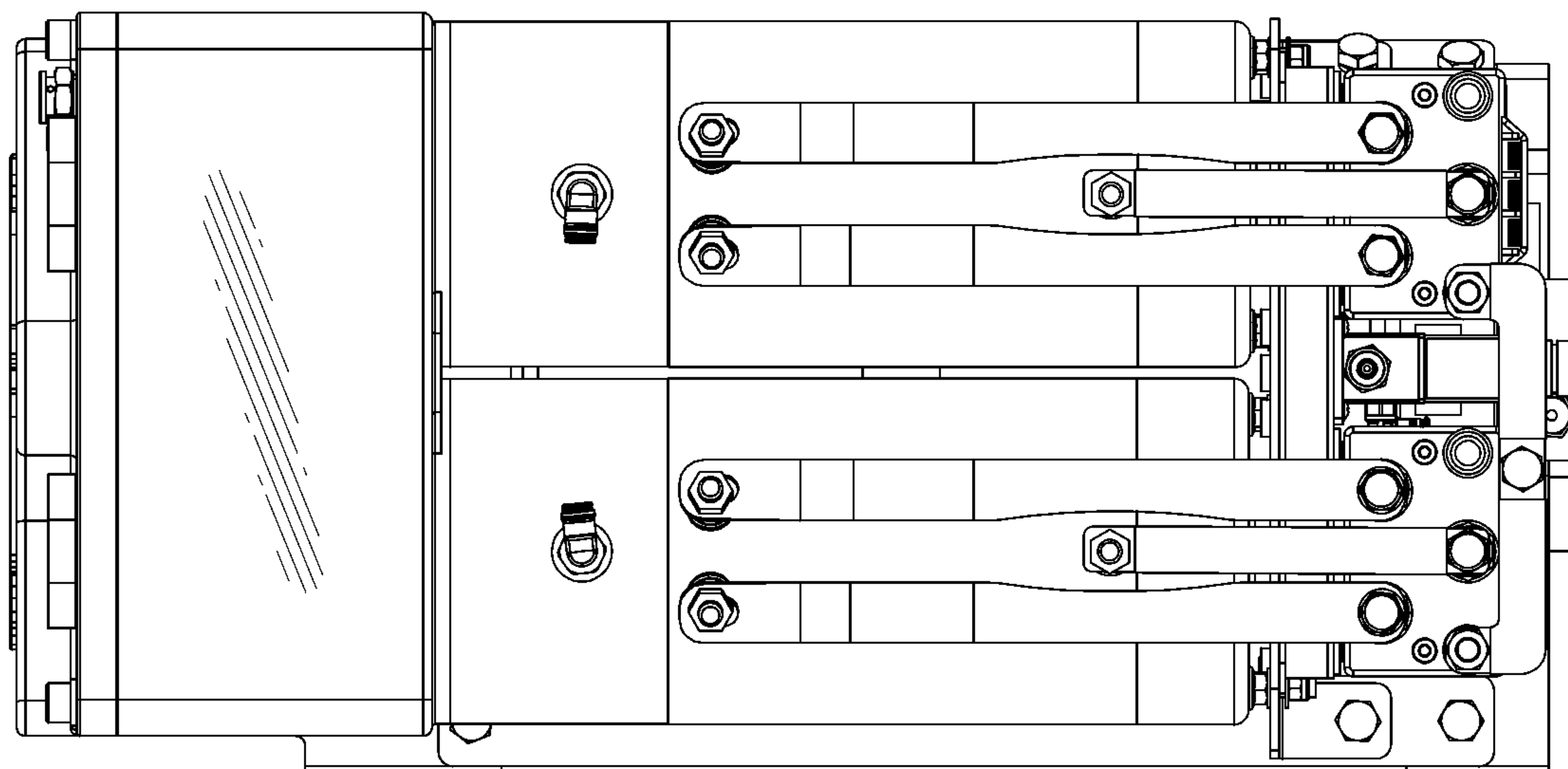
俯視圖
