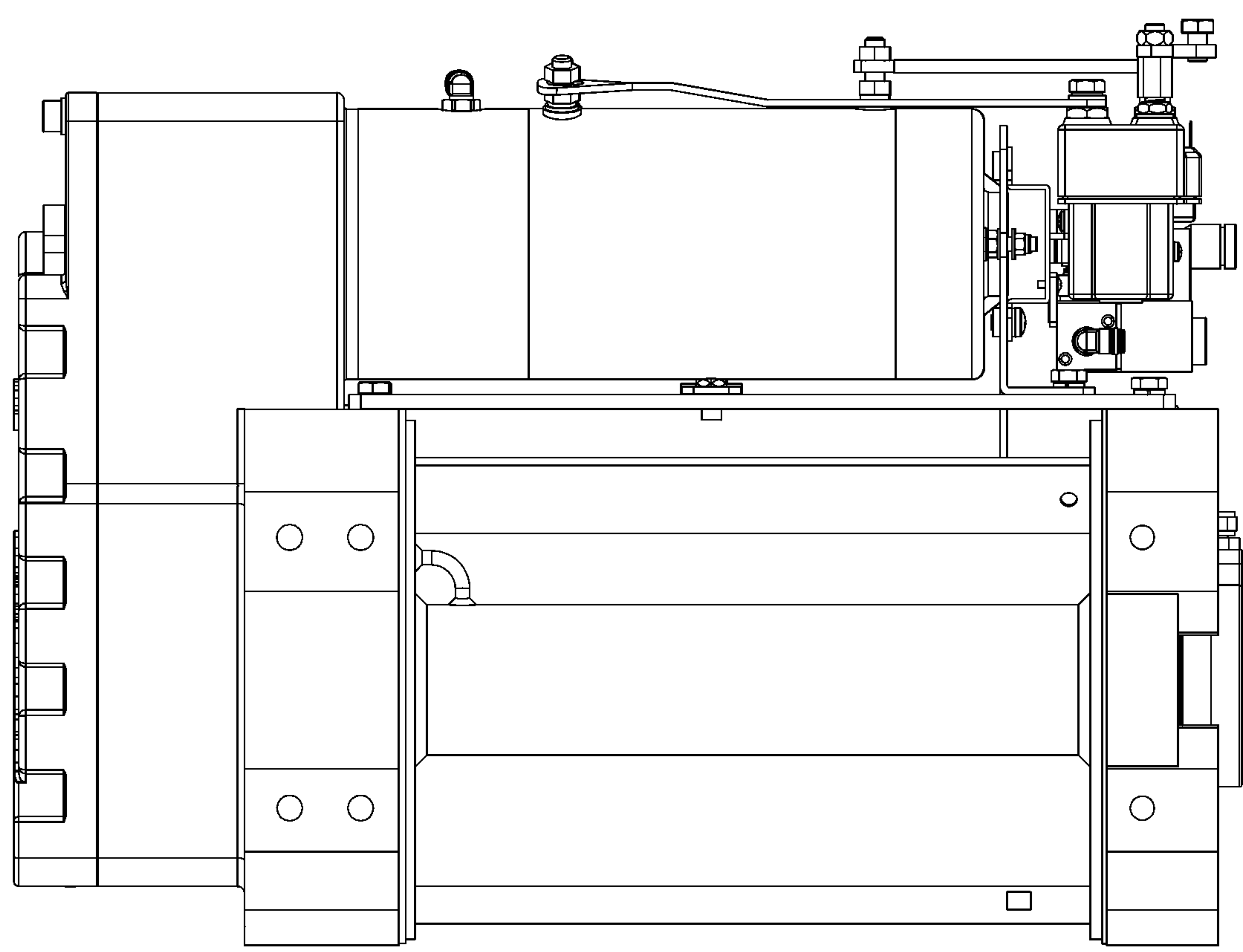
前視圖
