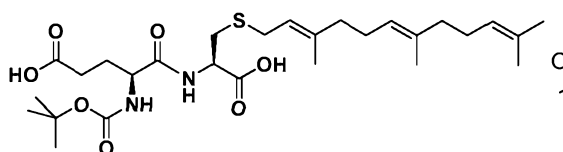
N-66;
