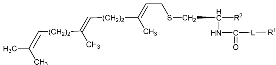
Ia
