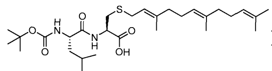
N-58
