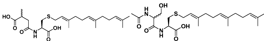
N-22;
