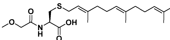
N-11;
