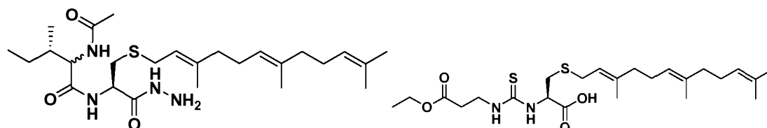
N-72;
