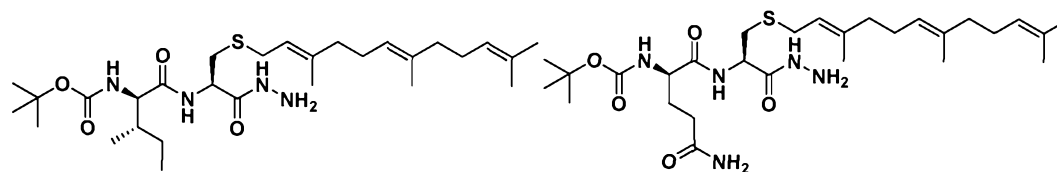
N-90;
