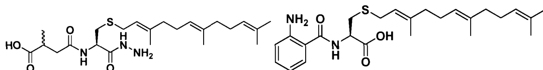
N-34;
