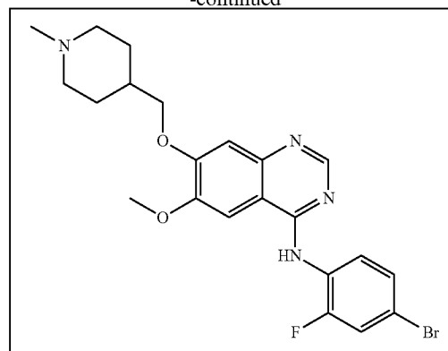
vandetanib
