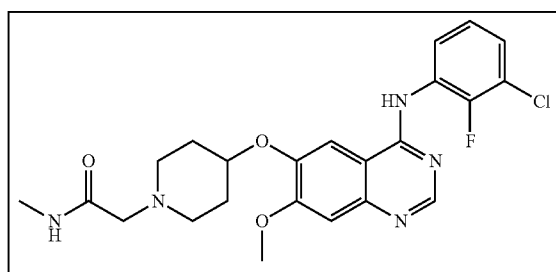
sapitinib
