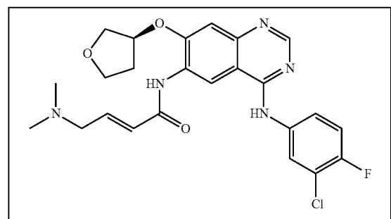
afatinib
