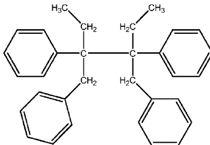
und 3,4-Dibenzyl-3,4-diphenylhexan (Struktur VIII)
