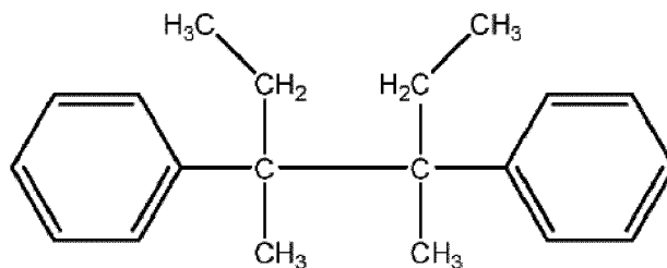
3,4-diéthyl-3,4-diphényl hexane (Structure IV)
