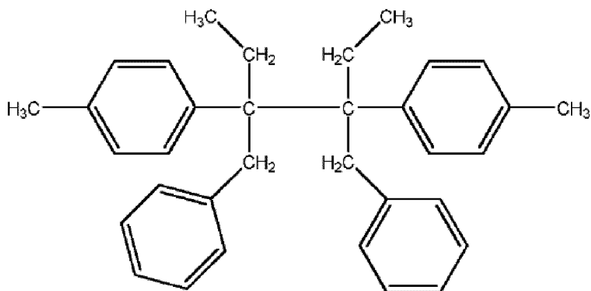
3,4-Dibenzyl-3,4-ditolylhexan (DBnDTH) (Struktur VI)
