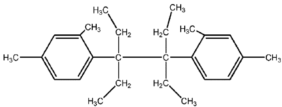
et 3,4-dibenzyl-3,4-diphényl hexane (Structure VIII)
