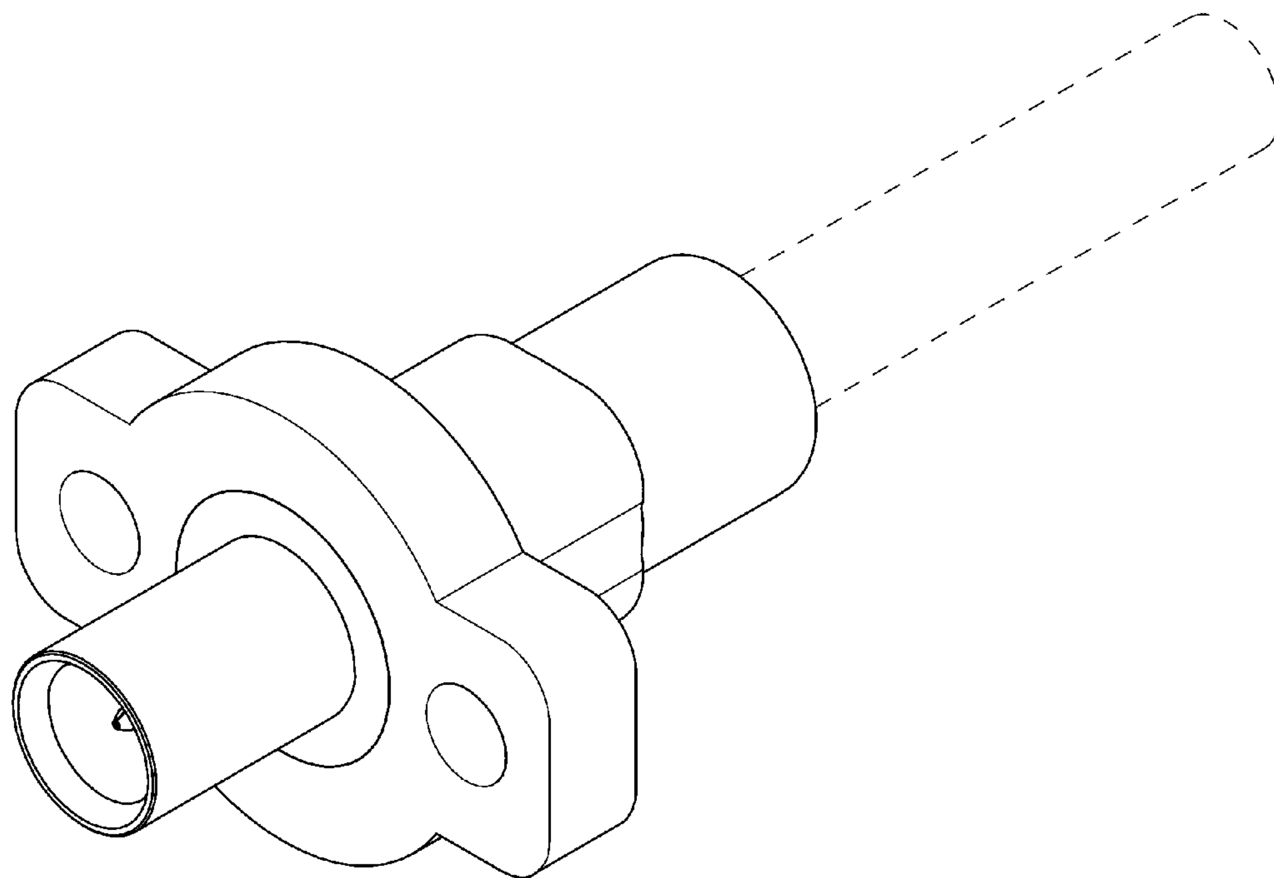
【立體圖 1】
