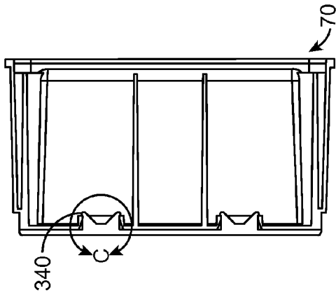
SECTION A-A FIG. 8C
