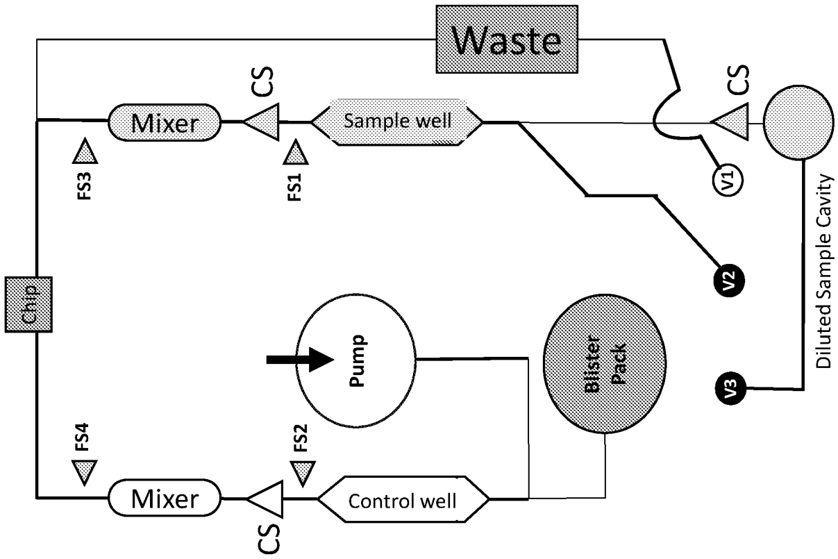
FIG. 20L (Empty control)
