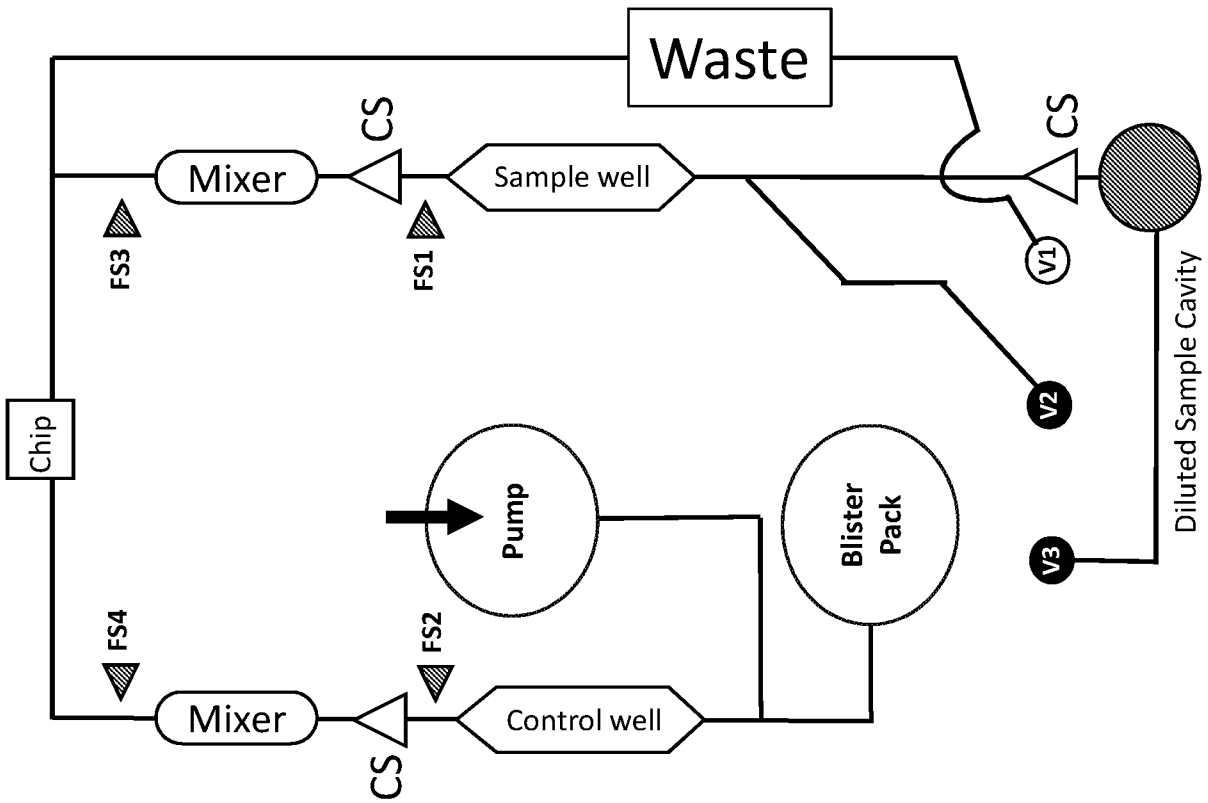
FIG. 20C (Prime pump)
