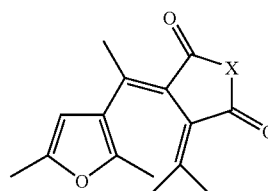
Fulgides (X = O) Fulgimides (X = NR)
