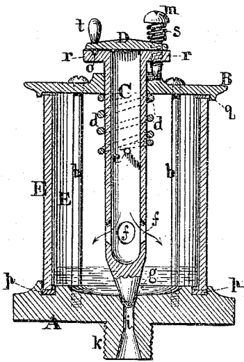
Fig. 1. (vert. sec.)
