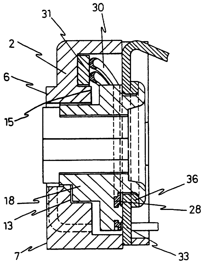
FIG. 3 B-B
