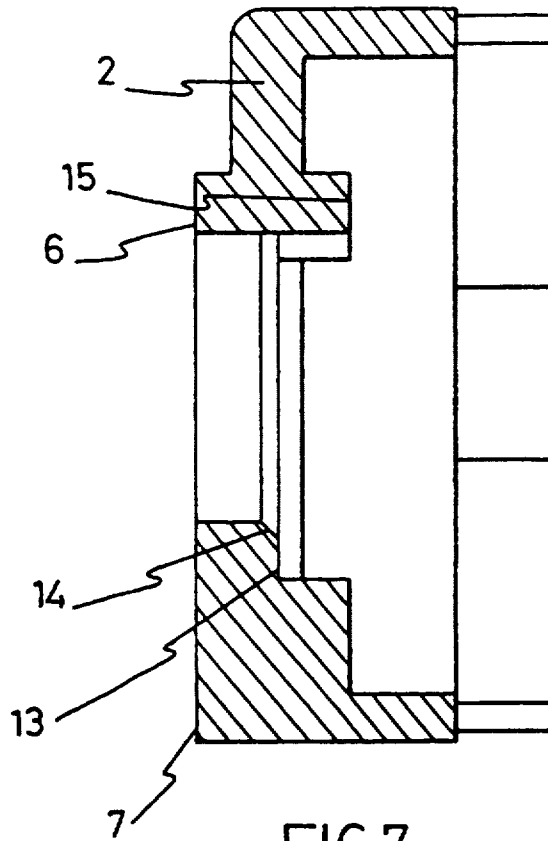
FIG. 7 C-C
