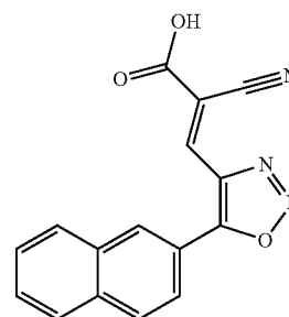
(E)-2-cyano-3-(5-(naphthalen-2-yl)-1,2,3-oxadiazol-4-yl)acrylic acid
