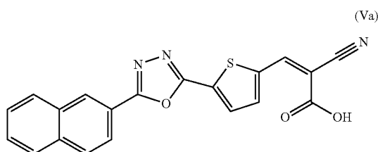
(Z)-2-cyano-3-(5-(5-(naphthalen-2-yl)-1,3,4-oxadiazol-2-yl)thiophen-2-yl)acrylic acid
