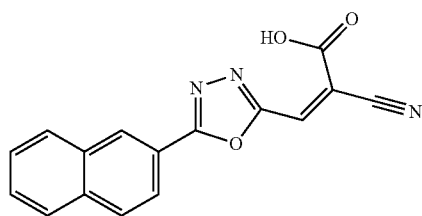
(Z)-2-cyano-3-(5-(naphthalen-2-yl)-1,3,4-oxadiazol-2-yl)acrylic acid
