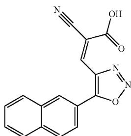
(Z)-2-cyano-3-(5-(naphthalen-2-yl)-1,2,3-oxadiazol-4-yl)acrylic acid
