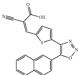
(Z)-2-cyano-3-(5-(5-(naphthalen-2-yl)-1,2,3-oxadiazol-4-yl)thiophen-2-yl)acrylic acid
