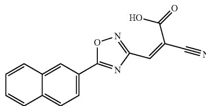
(Z)-2-cyano-3-(5-(naphthalen-2-yl)-1,2,4-oxadiazol-3-yl)acrylic acid
