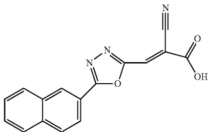
(E)-2-cyano-3-(5-(naphthalen-2-yl)-1,3,4-oxadiazol-2-yl)acrylic acid
