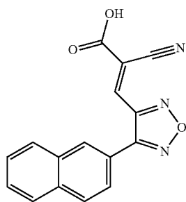
(E)-2-cyano-3-(4-(naphthalen-2-yl)-1,2,5-oxadiazol-3-yl)acrylic acid
