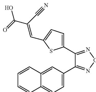
(E)-2-cyano-3-(5-(4-(naphthalen-2-yl)-1,2,5-oxadiazol-3-yl)thiophen-2-yl)acrylic acid
