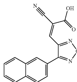
(Z)-2-cyano-3-(4-(naphthalen-2-yl)-1,2,5-oxadiazol-3-yl)acrylic acid
