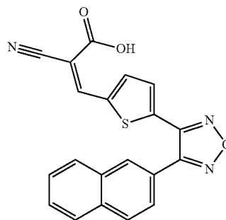
(Z)-2-cyano-3-(5-(4-(naphthalen-2-yl)-1,2,5-oxadiazol-3-yl)thiophen-2-yl)acrylic acid
