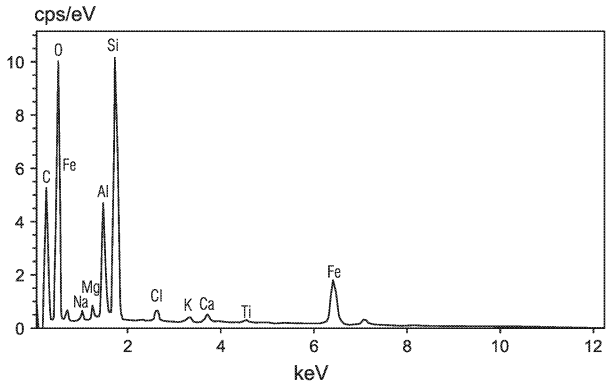
FIG. 8B
