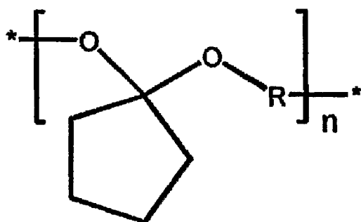
Poly(ortho esters)
