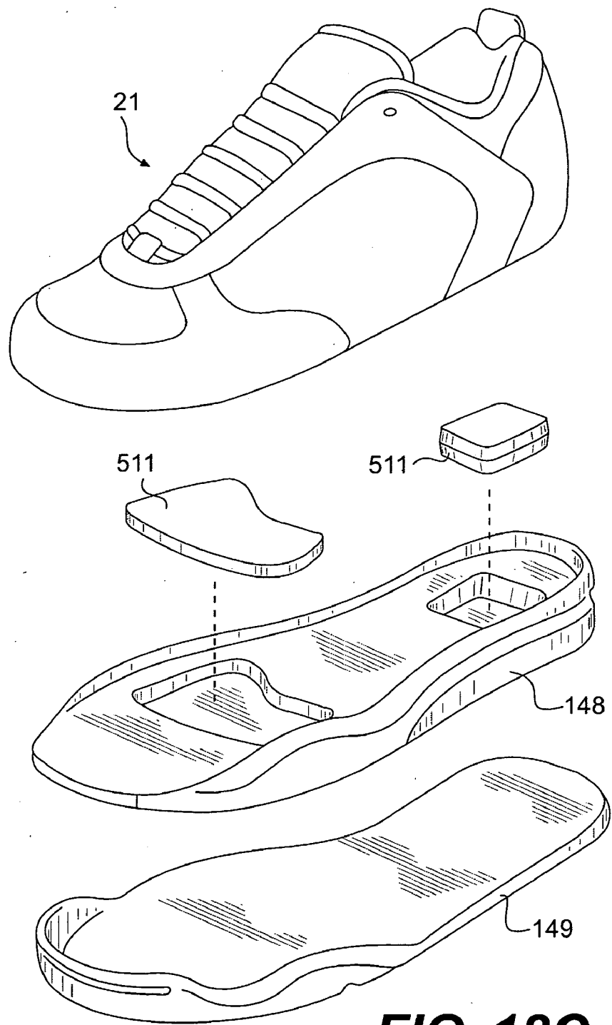
FIG. 18C
