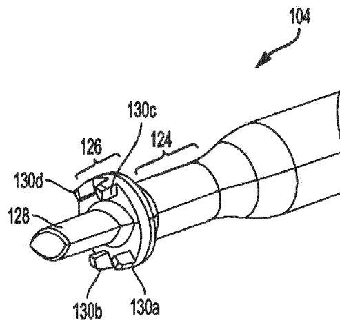
FIG. 4E
