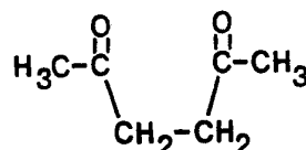
2,5-hexanedione
