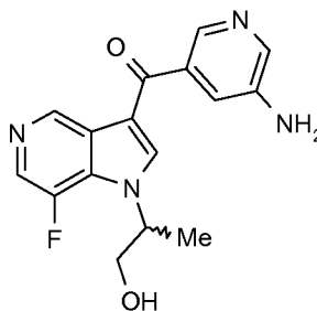
Enantiomer 2
