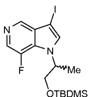
Enantiomer 1
