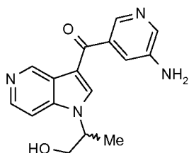
Enantiomer 1
