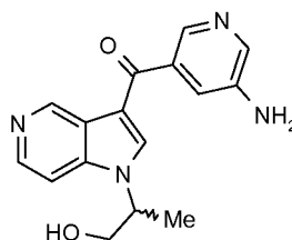
Enantiomer 2
