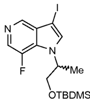
Enantiomer 2
