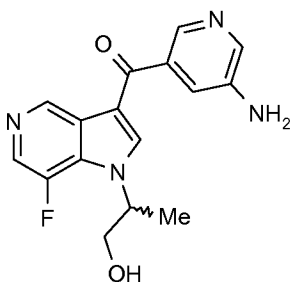
Enantiomer 1
