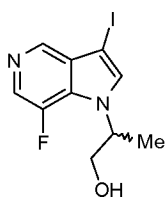
Enantiomer 1
