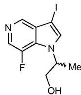
Enantiomer 2
