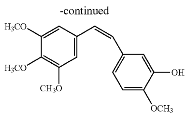
Combretastatin A-4
