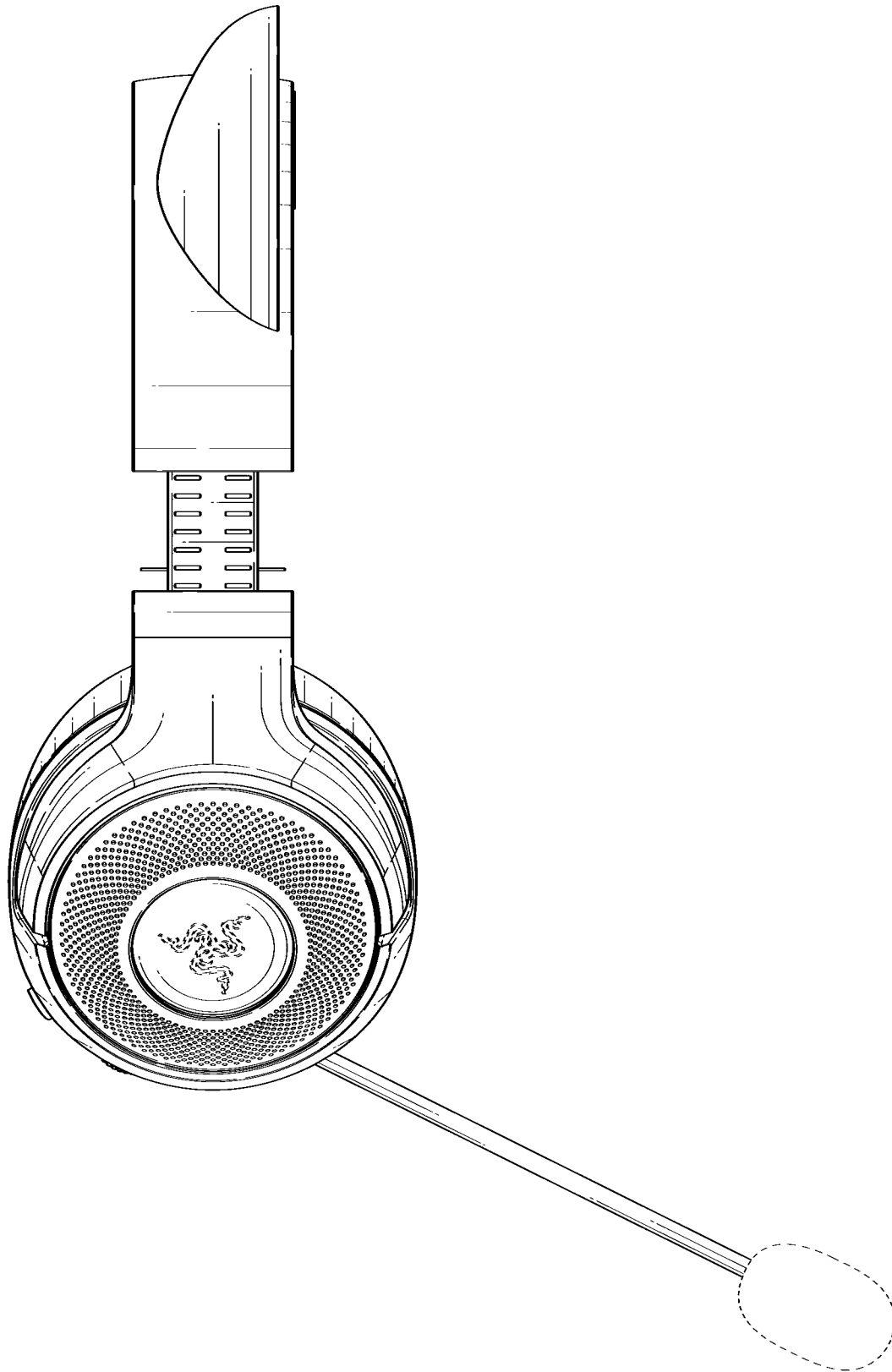
左側視圖
