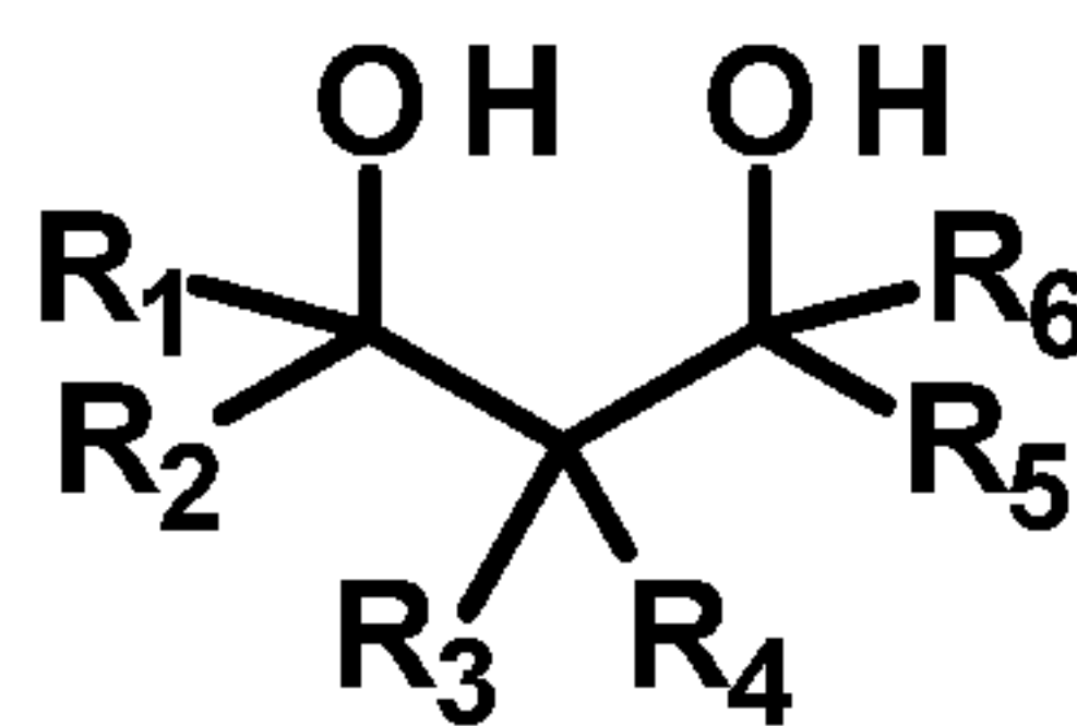
(III)
