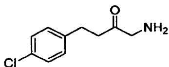
1-amino-4-(4-chlorophenyl)butan-2-one
