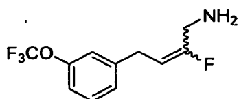
2-fluoro-4-(3-(trifluoromethoxy)phenyl)but-2-en-1-amine
