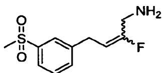
2-fluoro-4-(3-(methylsulfonyl)phenyl)but-2-en-1-amine
