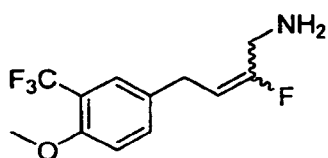
2-fluoro-4-(4-methoxy-3-(trifluoromethyl)phenyl)but-2-en-1-amine
