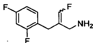
2-(2,4-difluorobenzyl)-3-fluoroprop-2-en-1-amine
