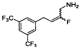
4-(3,5-bis(trifluoromethyl)phenyl)-2-fluorobut-2-en-1-amine
