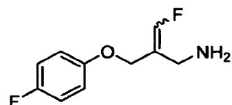
3-fluoro-2-((4-fluorophenoxy)methyl)prop-2-en-1-amine
