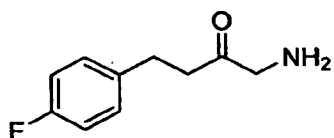
1-amino-4-(4-fluorophenyl)butan-2-one
