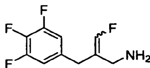
3-fluoro-2-(3,4,5-trifluorobenzyl)prop-2-en-1-amine
