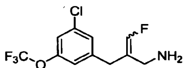
2-(3-chloro-5-(trifluoromethoxy)benzyl)-3-fluoroprop-2-en-1-amine
