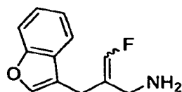
2-(benzofuran-3-ylmethyl)-3-fluoroprop-2-en-1-amine
