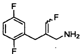
2-(2,5-difluorobenzyl)-3-fluoroprop-2-en-1-amine
