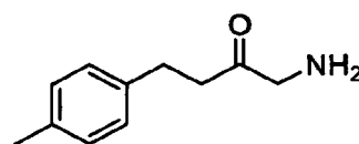
1-amino-4- p -tolylbutan-2-one
