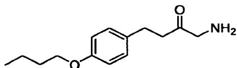
1-amino-4-(4-butoxyphenyl)butan-2-one
