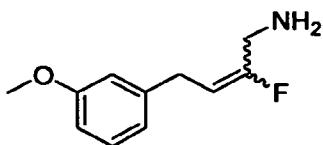
2-fluoro-4-(3-methoxyphenyl)but-2-en-1-amine
