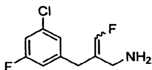
2-(3-chloro-5-fluorobenzyl)-3-fluoroprop-2-en-1-amine
