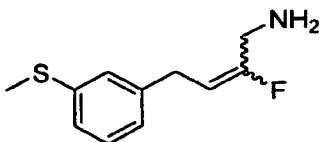
2-fluoro-4-(3-(methylthio)phenyl)but-2-en-1-amine
