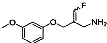
3-fluoro-2-((3-methoxyphenoxy)methyl)prop-2-en-1-amine
