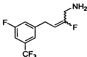
2-fluoro-4-(3-fluoro-5-(trifluoromethyl)phenyl)but-2-en-1-amine
