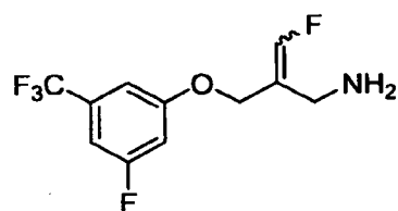
3-fluoro-2-((3-fluoro-5-(trifluoromethyl)phenoxy)methyl)prop-2-en-1-amine
