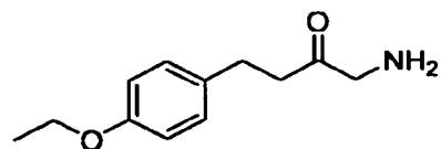
1-amino-4-(4-ethoxyphenyl)butan-2-one
