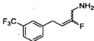
2-fluoro-4-(3-(trifluoromethyl)phenyl)but-2-en-1-amine
