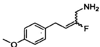
2-fluoro-4-(4-methoxyphenyl)but-2-en-1-amine
