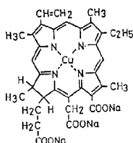
Chlorophyllin
