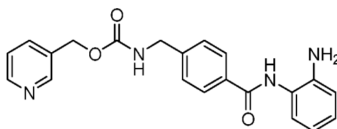
MS-275
