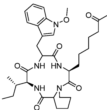
Apicidin
