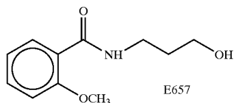
3-(2-methoxybenzoylamino)-1-propanol
