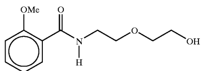
2-[2-N-(2-methoxybenzoyl)aminoethoxy]ethanol
