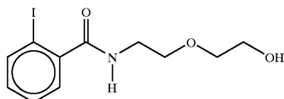
2-[N-(2-iodobenzoyl)aminoethoxy]ethanol
