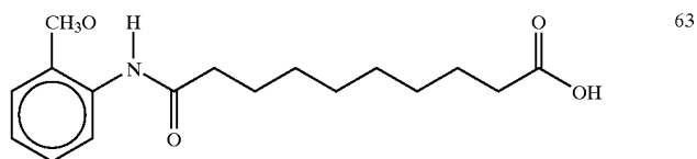
10-(N-2-Methoxyanilino)sebalic acid
