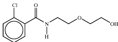
2-[2-N-(2-chlorobenzoyl)aminoethoxy]ethanol
