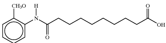
10-(N-2-Methoxyanilino)sebalic acid
