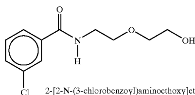
2-[2-N-(3-chlorobenzoyl)aminoethoxy]ethanol
