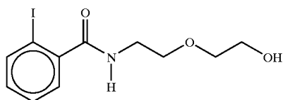
2-[N-(2-iodobenzoyl)aminoethoxy]ethanol
