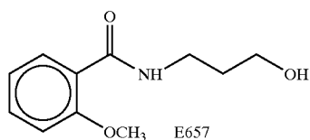
3-(2-methoxybenzoylamino)-1-propanol
