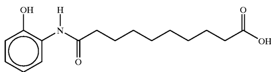
10-(N-2-Methoxyanilino)sebalic acid
