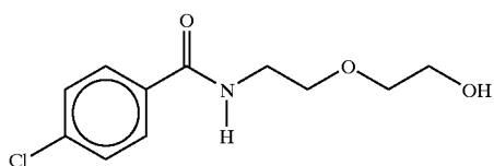
2-[2-N-(4-chlorobenzoyl)aminoethoxy]ethanol
