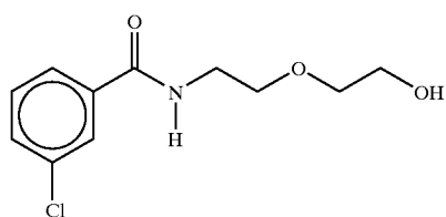
2-[2-N-(3-chlorobenzoyl)aminoethoxy]ethanol
