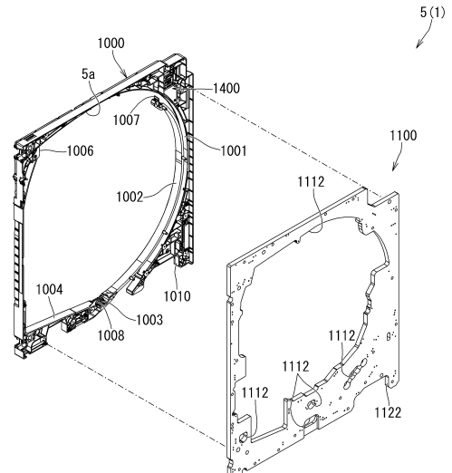
【図 1 3 0】
